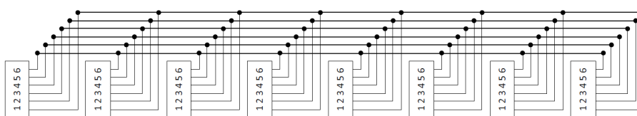
Схема подключения KP-124
