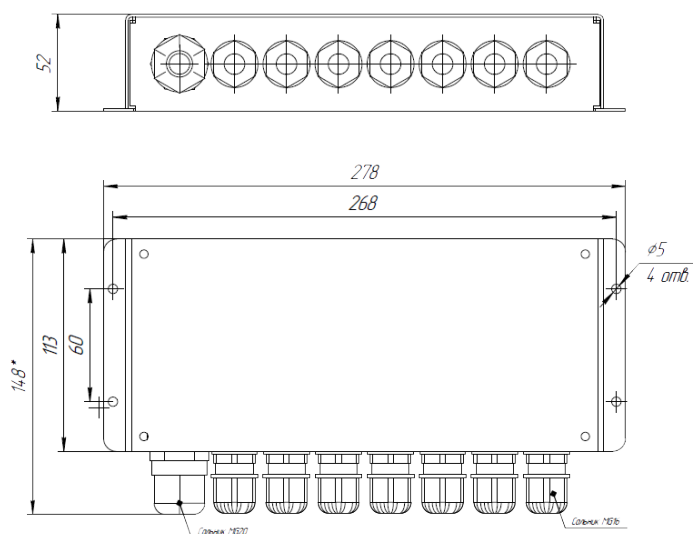
Габаритные и установочные размеры KP-124 (S, P)
