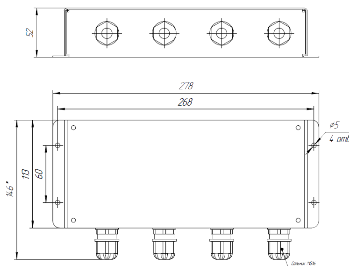
Габаритные и установочные размеры KP-124
